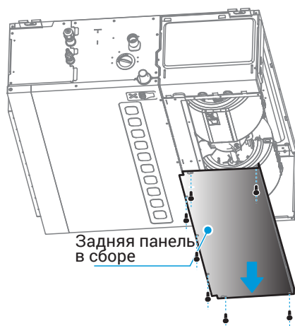
Демонтаж задней панели
