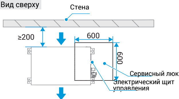
Вид сверху
