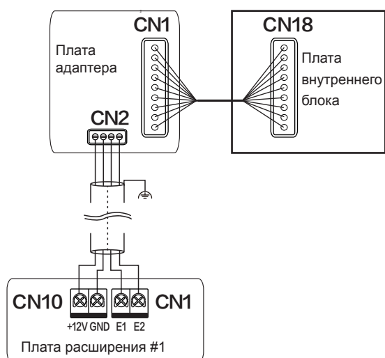
Только плата расширения #1
