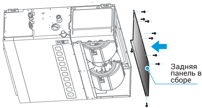
Монтаж задней панели
