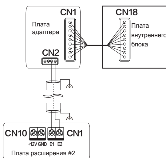
Только плата расширения #2
