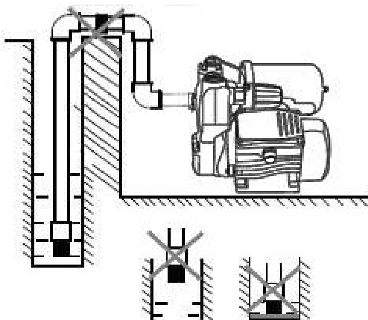
Неправильная установка.
