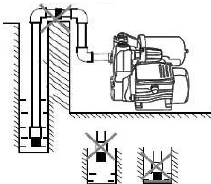
Неправильная установка.
