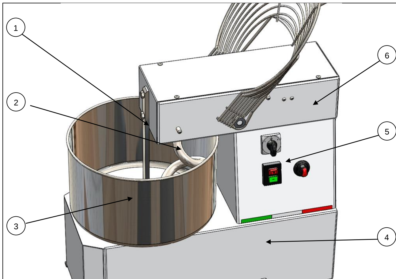
Рисунок 3-1 Схема машины
