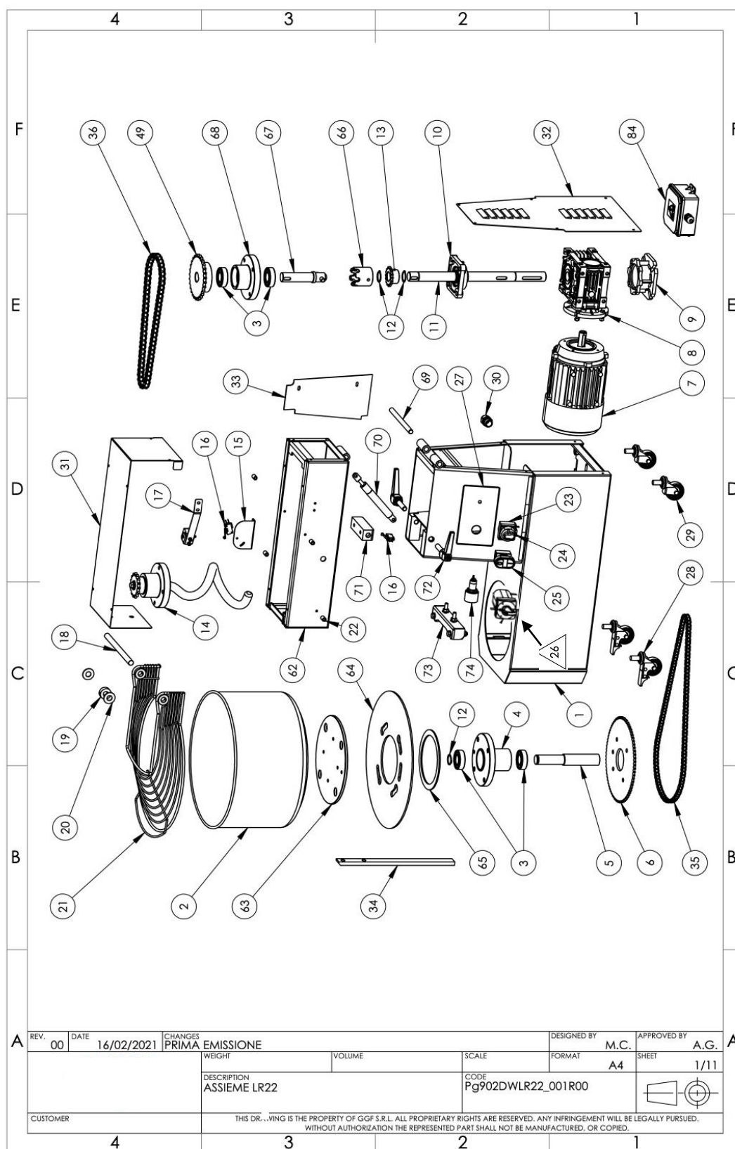
Figura 10-20. сборка LR22 / LR33 / LR42
