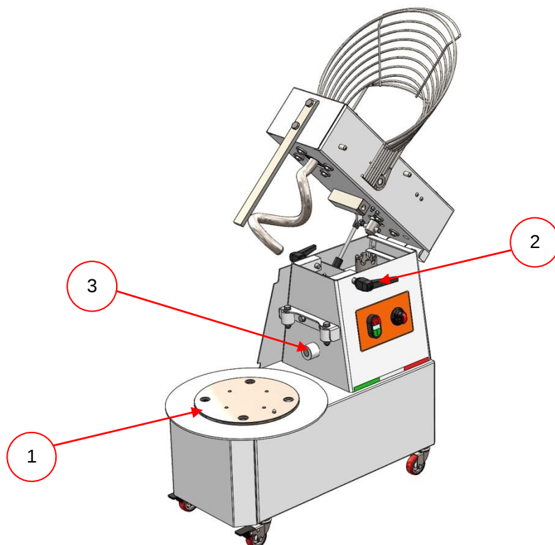
Figura 3-2 ТЕСТОМЕСИЛЬНАЯ МАШИНА LR
